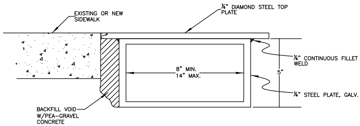
SEC-"A-A"
